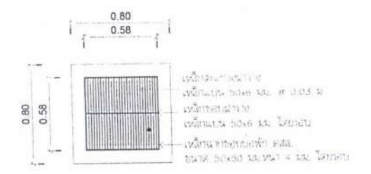
แบบขยายตามภาพท่อ คลัง มาตราส่วน 1 : 30
