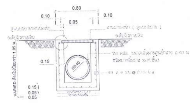
แบบรูปตัด (๑) - (๑) มาตราส่วน 1 : 30
