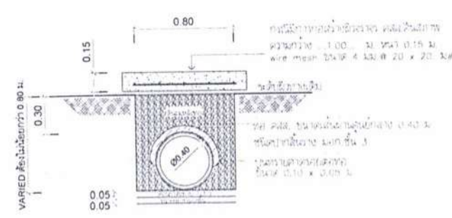
แบบรูปตัด (๒) - (๒) มาตราส่วน 1 : 30
