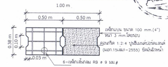
ขยายขอบราง
