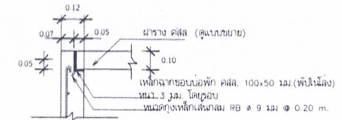
ขยายขอบราง คสล.
