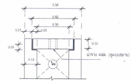
แบบขยายระบายน้ำราง คสล.
