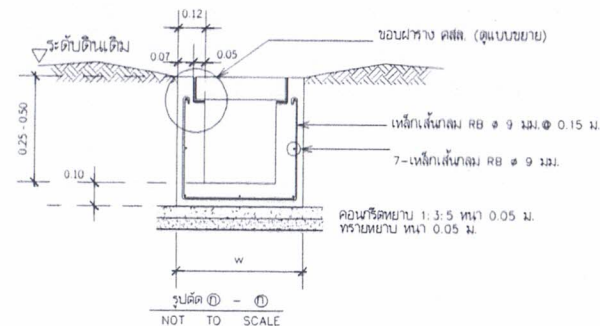
แปลร่างระบายน้ำราง คสล.
