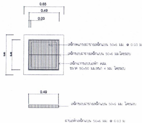
แบบขยายจากภาพเหล็ก คลส. มาตราส่วน 1 : 30
